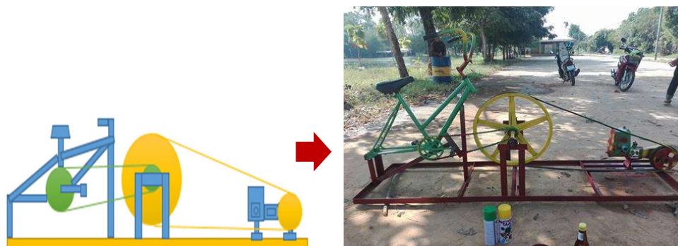
ภาพที่ 1 ร่างแบบฐานจักรยาน และส่วนประกอบที่สร้างจริง
