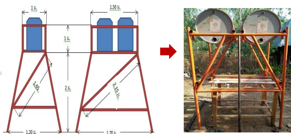
ภาพที่ 2 ร่างแบบฐานของถังพักน้ำและส่วนประกอบที่สร้างจริง
