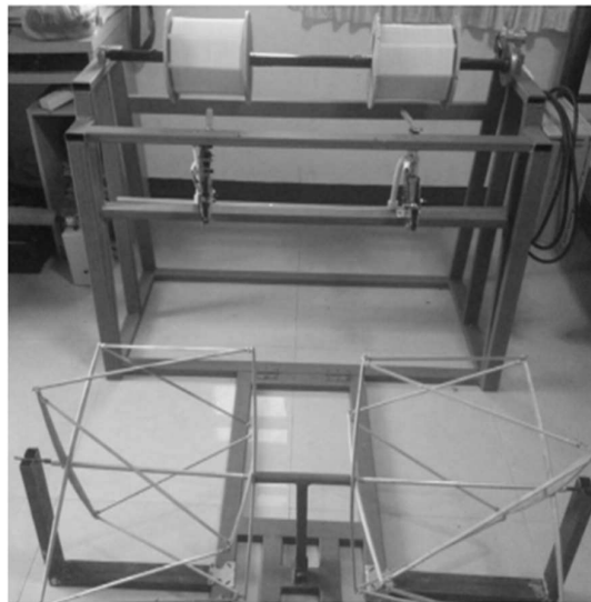
ภาพที่ 4 การออกแบบสร้างเครื่องกรอด้ายไฟฟ้า
