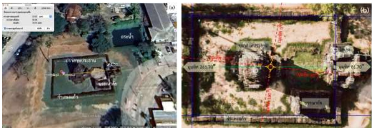
รูปที่ 5 (a) การวัดมุมทิศของปรางค์กู่ชัยภูมิโดยใช้โปรแกรมแผนที่อิเล็กทรอนิกส์ (b) การเบี่ยงจากแกนทิศตะวันออกแท้ของปรางค์กู่ชัยภูมิ
