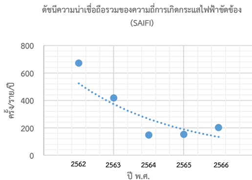
Figure 2 ดัชนีความน่าเชื่อถือรวมของความเสี่ยงการเกิดกระแสไฟฟ้าขัดข้อง
